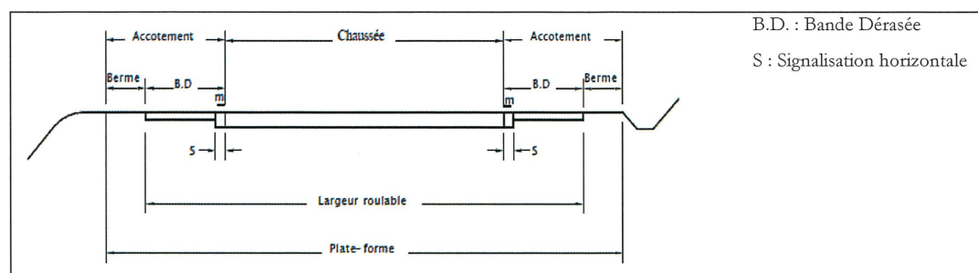
Figure 1 – Schéma de principe d'une plate-forme de route bidirectionnelle (Rosey & Moisan, 2011, p.13). La plate-forme est un des éléments du profil en travers, et c'est la surface de la route qui comprend la ou les chaussée(s), les accotements et le terre-plein éventuel (Setra, 2006), et des pistes spéciales éventuelles pour piétons et cyclistes (Accord Européen Grandes Routes, 2008).
